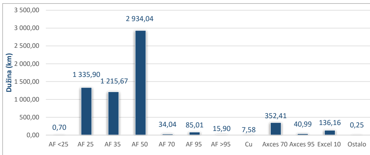
Slika 20 Dužine 10 i 20 kV nadzemnih vodova prema materijalu i presjeku vodiča
