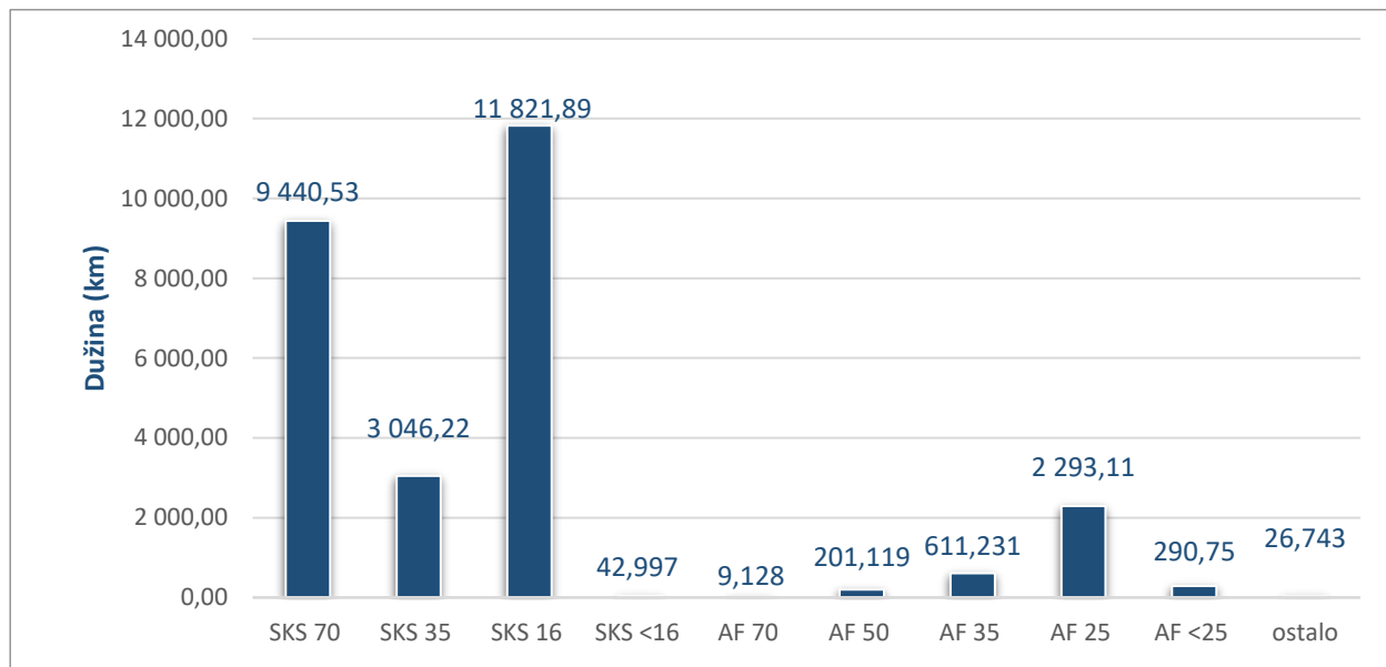
Slika 23 Pregled niskonaponske nadzemne mreže prema izvedbi i presjeku vodiča
