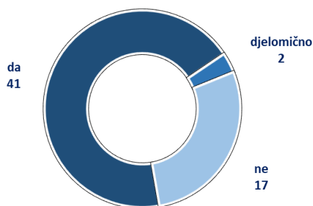
Slika 11 Pregled pripremljenosti SN postrojenja za pogonski napon 20 kV u TS 110/x kV
